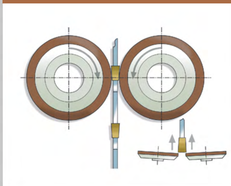
Заточка боковой грани
